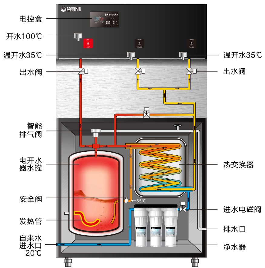
(碧丽常压式节能饮水机专利原理图)
