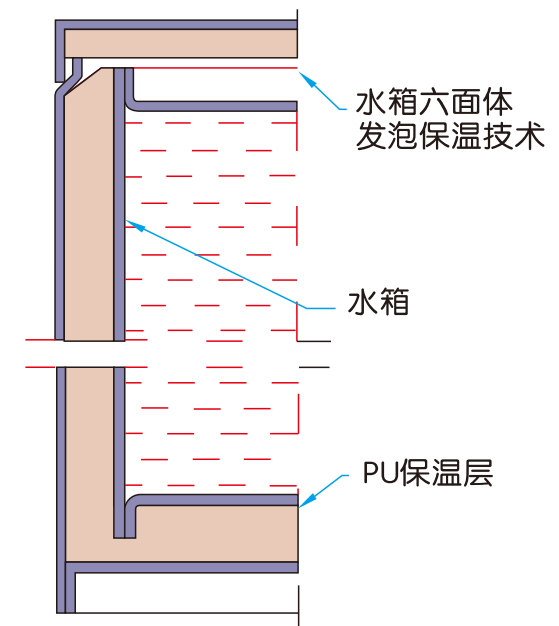
图3碧丽六面体保温结构图
