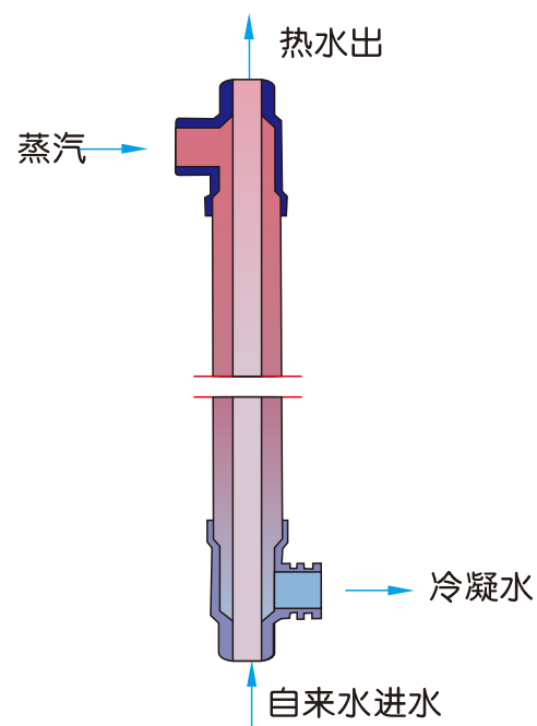
图2蒸汽冷凝装置图
