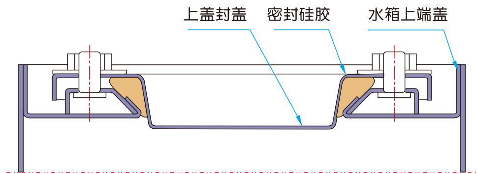
图1内胆上端盖密封方式
